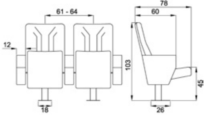
Estructura de asiento metálica / Posavasos integrados / Asiento tapizado / Numeración butaca bordada / Numeración de fila en chapa de metacrilato Metal seat structure / Integrated cupholders / Upholstered seat / Embroidered seat numbering / Row numbering on methacrylate sheet Structure de siège en métal / Porte-gobelets intégrés / Siège rembourré / Numérotation des sièges brodés / Numérotation bout de rangée acrylate Каркас сидения из металла / Встроенные подстаканники / Мягкое сидение / Вышитая нумерация кресел / Пластиковые номера рядов
