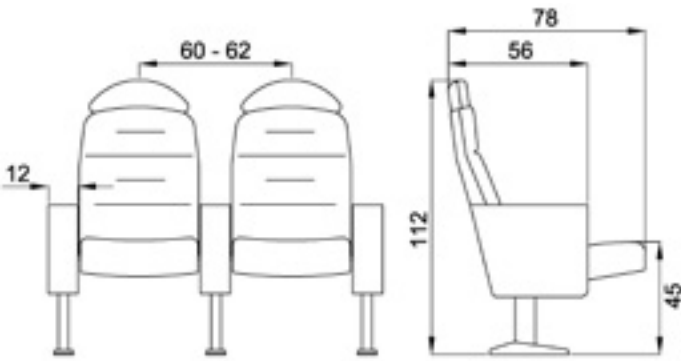
Reposacabezas / Compactos tapizados / Posavasos integrado / Numeración butaca bordada / Numeración de fila en consola de polipropileno Headrest / Upholstered panels / Integrated cupholders / Embroidered seat numbering / Row numbering on polypropylene console Appui-tête / Panneaux rembourrés / Porte-gobelets intégrés / Numérotation des sièges brodés / Numérotation des rangées par plaquette en polypropylène Подголовник / Панель в обивке / Встроенные подстаканники / Вышитая нумерация кресел / Нумерация рядов на пластиковых консолях
