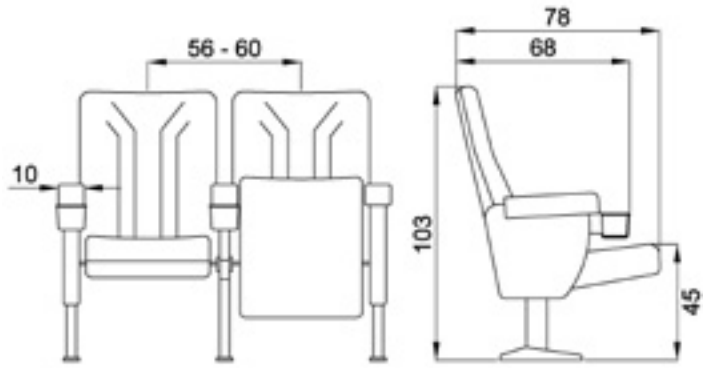
Estructura de asiento metálica / Posavasos de polipropileno / Apoyabrazos tapizados / Asiento tapizado Metal seat structure / Polypropylene cupholders / Upholstered armrests / Upholstered seat Structure de siège en métal / Porte-gobelets en polypropylène / Accoudoirs rembourrés / Siège rembourré Каркас сидения из металла / Полипропиленовые подстаканники / Подлокотники в обивке / Мягкое сидение
