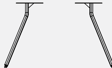
ODLA73 L 1218 mm W 536 mm H 730 mm 10,5 kg
