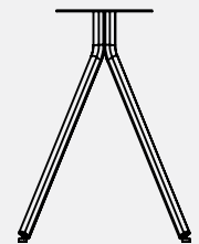
ODLA73 (una pata/ one leg) L 429 mm W 536 mm H 730 mm 5,2 kg
